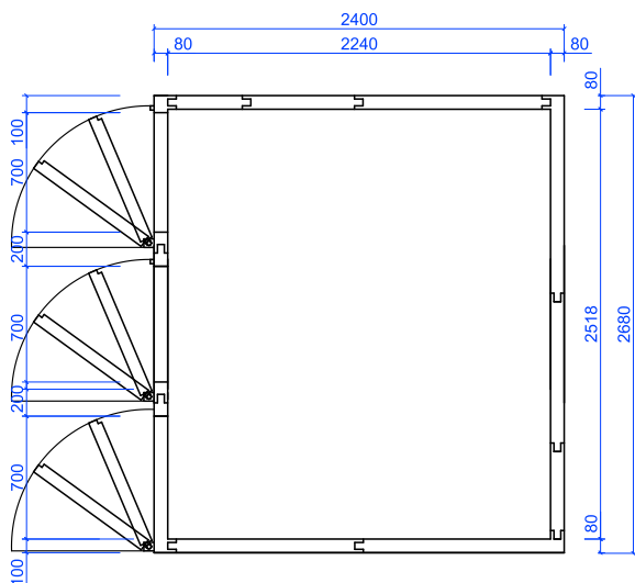
Standardní chladicí box QL 270
